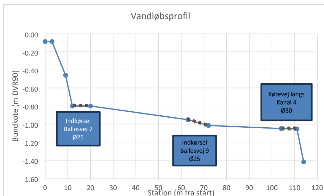
Figur 2. Vejgrøftens profil fra st. 0-114.
