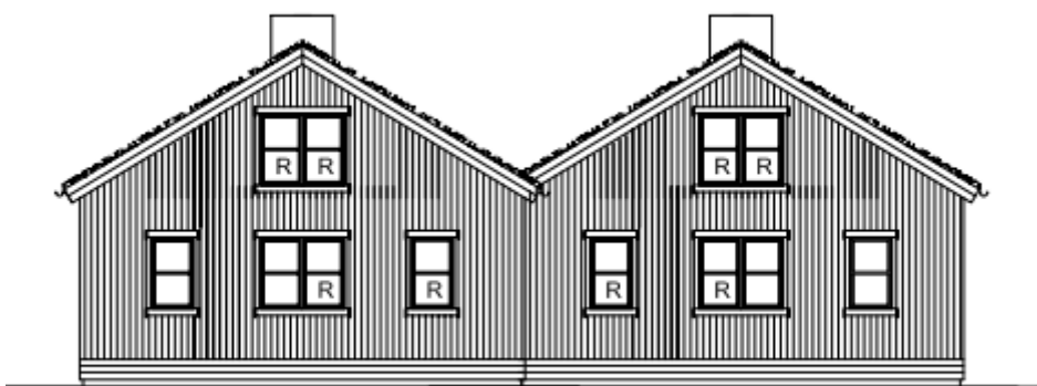
Nordfacade
