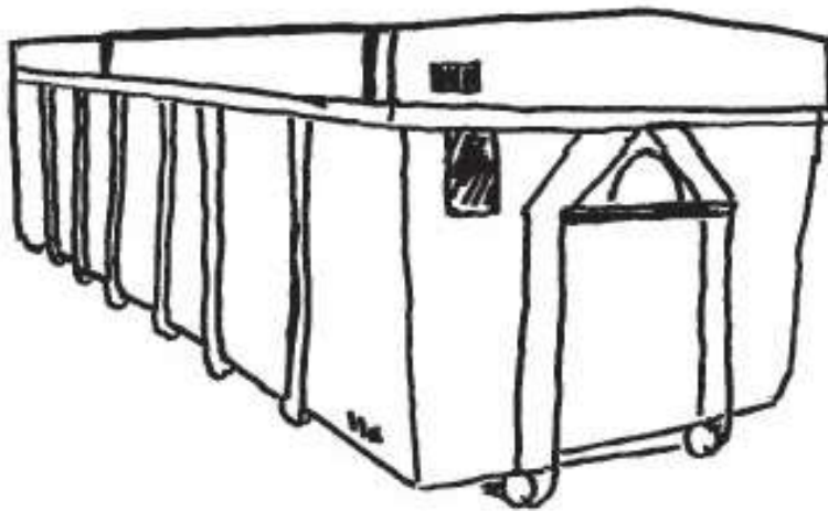
Eksempel på udendørs opbevaring af olieholdige metalspåner i dobbeltbundet container med skydelåg.
