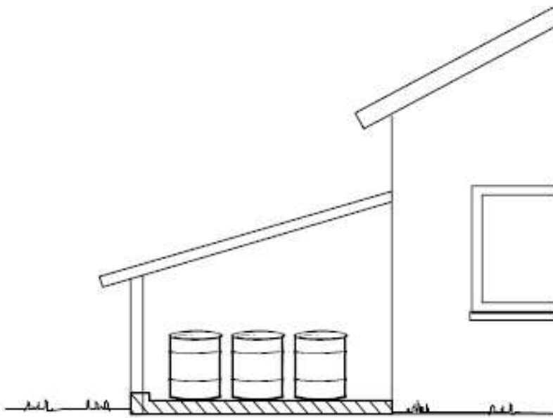
Overdækket plads med støbt betongulv med opkant som afgrænsning.
