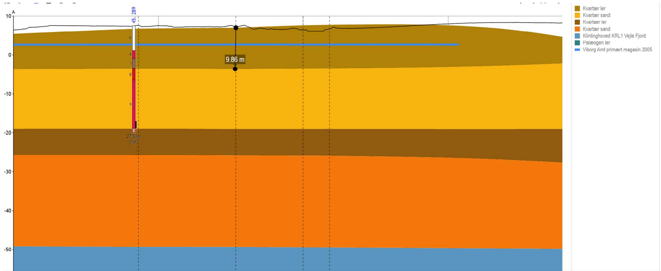
Bilag 2. Geologisk tværsnit fra GeoAtlas, der viser lagfølgen fra indvindingsboringerne via nedgravningsstedet til den § 3-beskyttede sø og videre mod kysten. Nedgravningsstedet er markeret ved den lodrette streg, der angiver lerlagets tykkelse.
