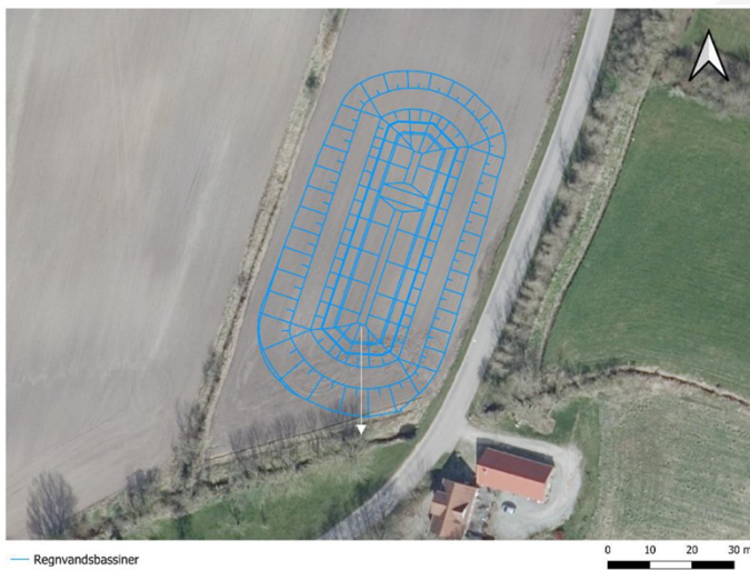
Figur 3 Udformningen af regnvandsbassinet ved matr.nr. 4d Sundby By, Sundby. Hvid pil indikerer udledningspunkt til Thorup-Skallerup Bæk
