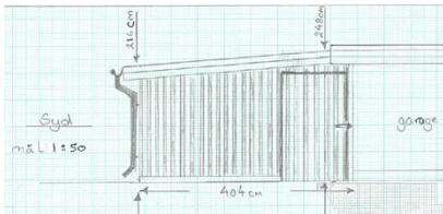
Fig. 3: Indsendt facadetegning
